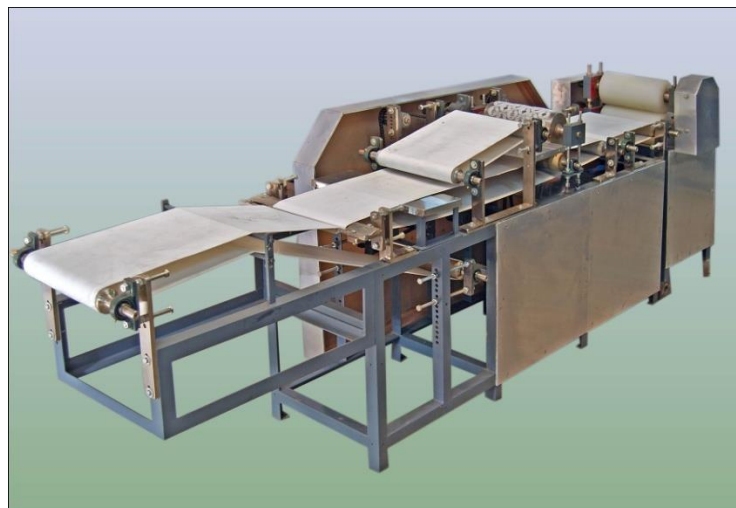
(2). Semi Auto Papad Machine Super Delux.
